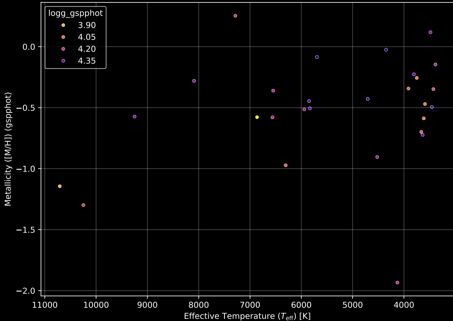
Gaia Cluster: [UPK_526] Stellar Population Parameters (n= 28)
