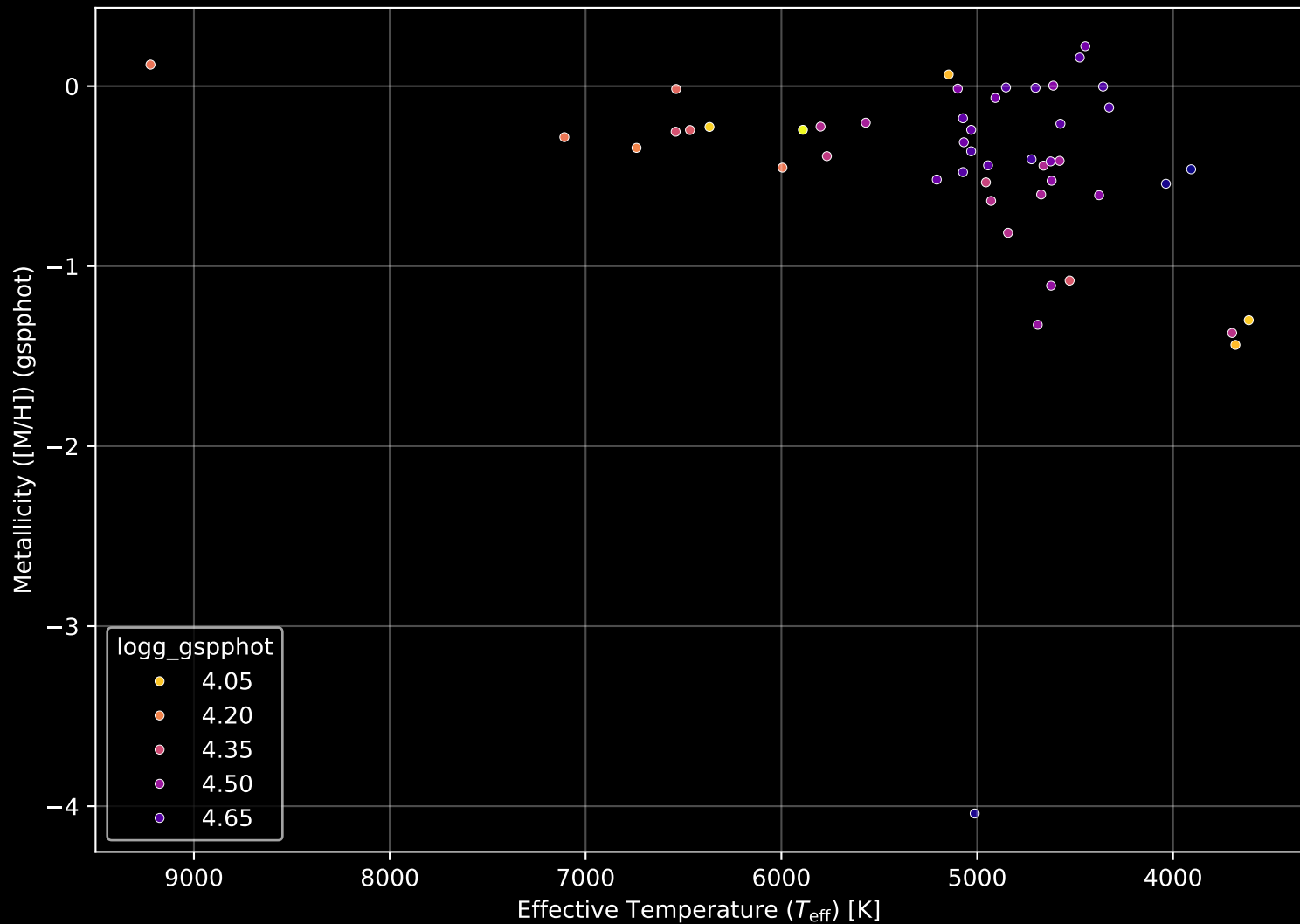
Gaia Cluster: [UPK_528] Stellar Population Parameters (n= 49)
