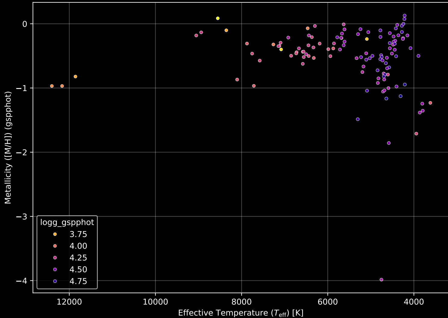
Gaia Cluster: [UPK_54] Stellar Population Parameters (n= 119)
