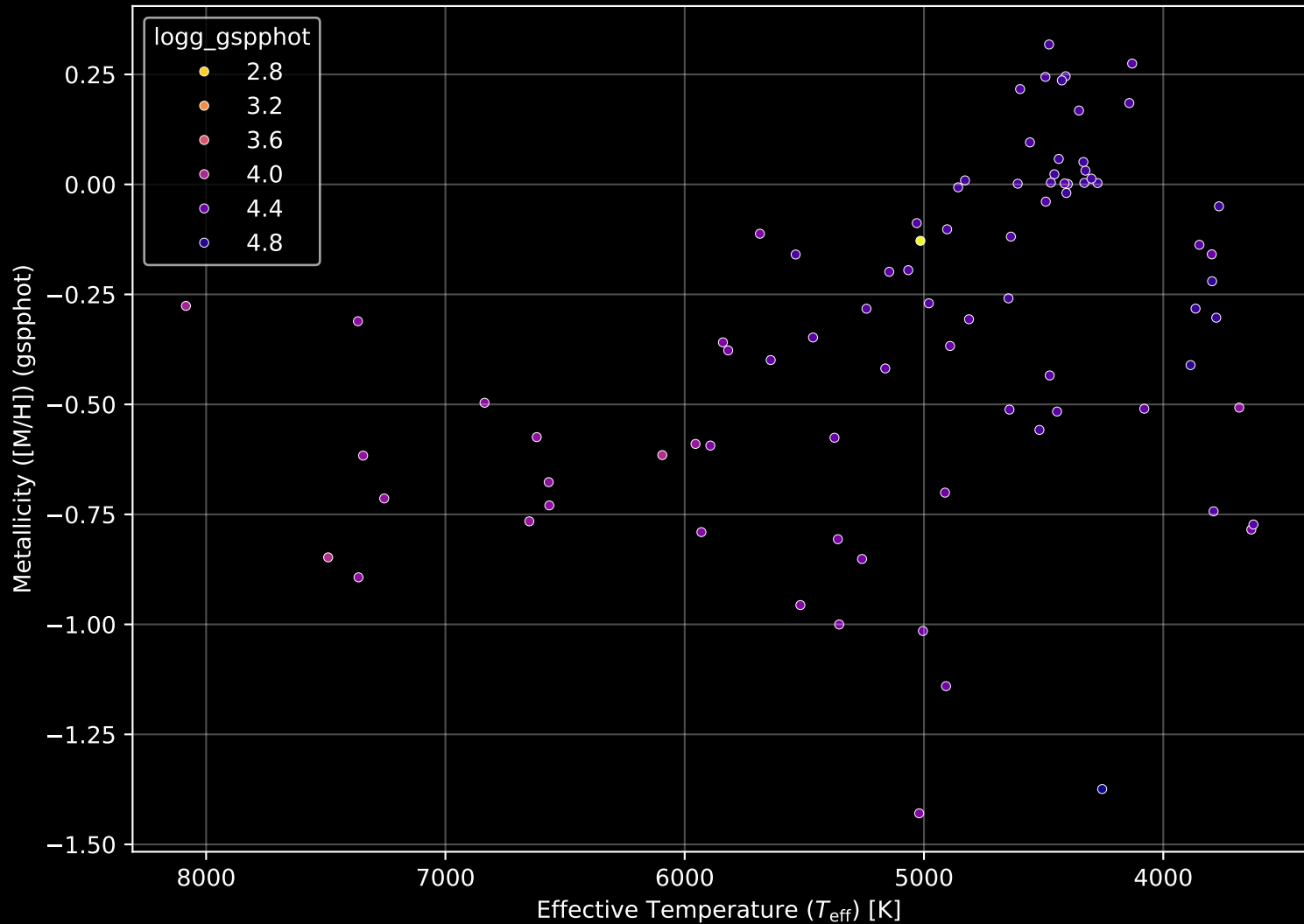
Gaia Cluster: [UPK_567] Stellar Population Parameters (n= 83)
