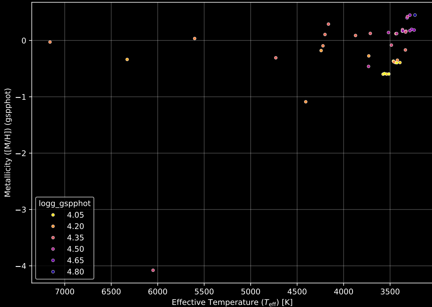
Gaia Cluster: [UPK 606] Stellar Population Parameters (n= 41)
