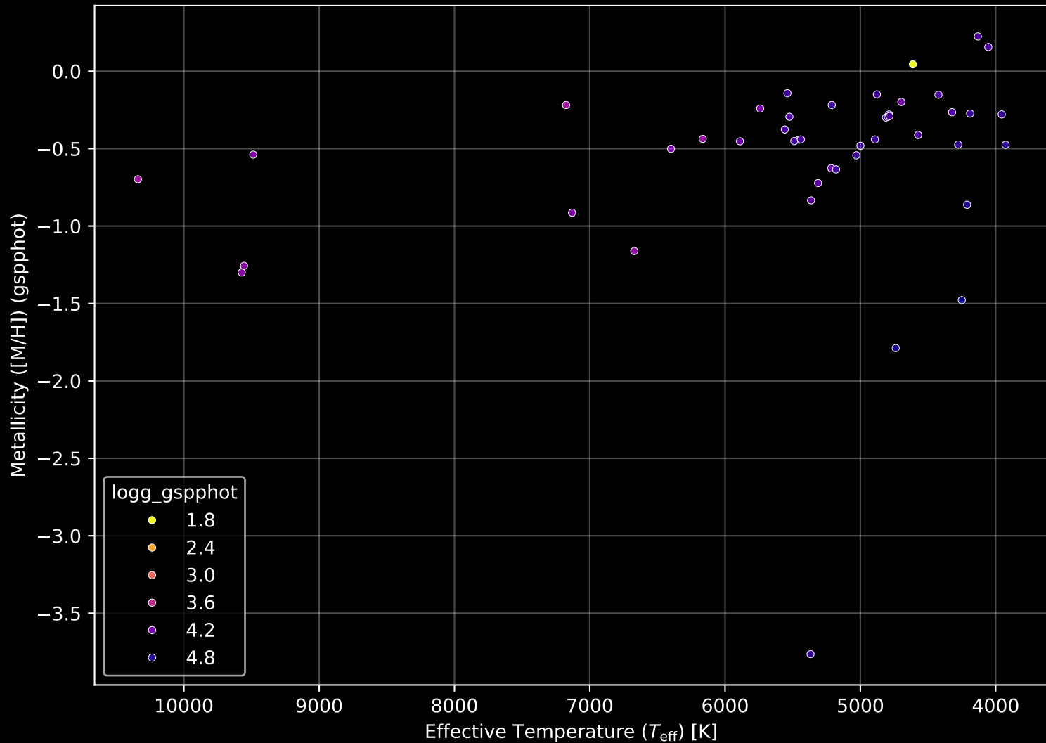
Gaia Cluster: [UPK_613] Stellar Population Parameters (n= 45)
