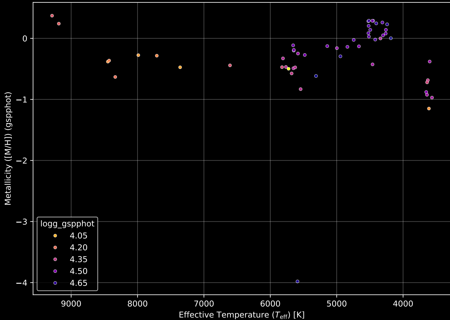
Gaia Cluster: [UPK_645] Stellar Population Parameters (n= 55)
