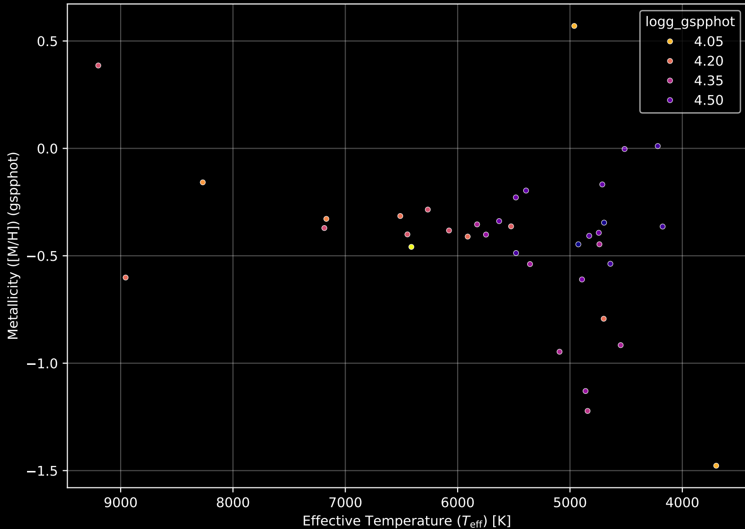
Gaia Cluster: [UPK_94] Stellar Population Parameters (n= 37)
