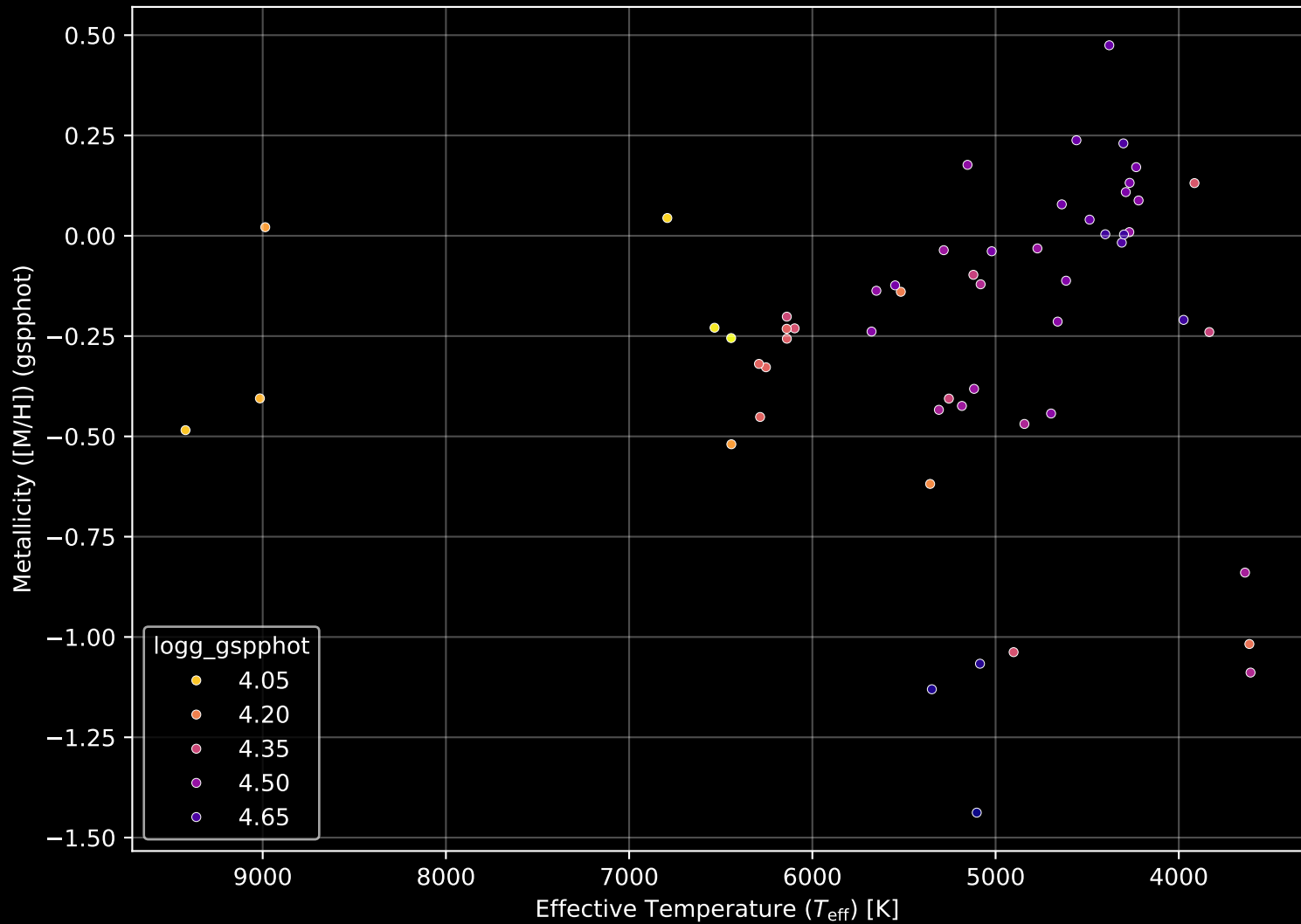
Gaia Cluster: [UPK_99] Stellar Population Parameters (n= 56)
