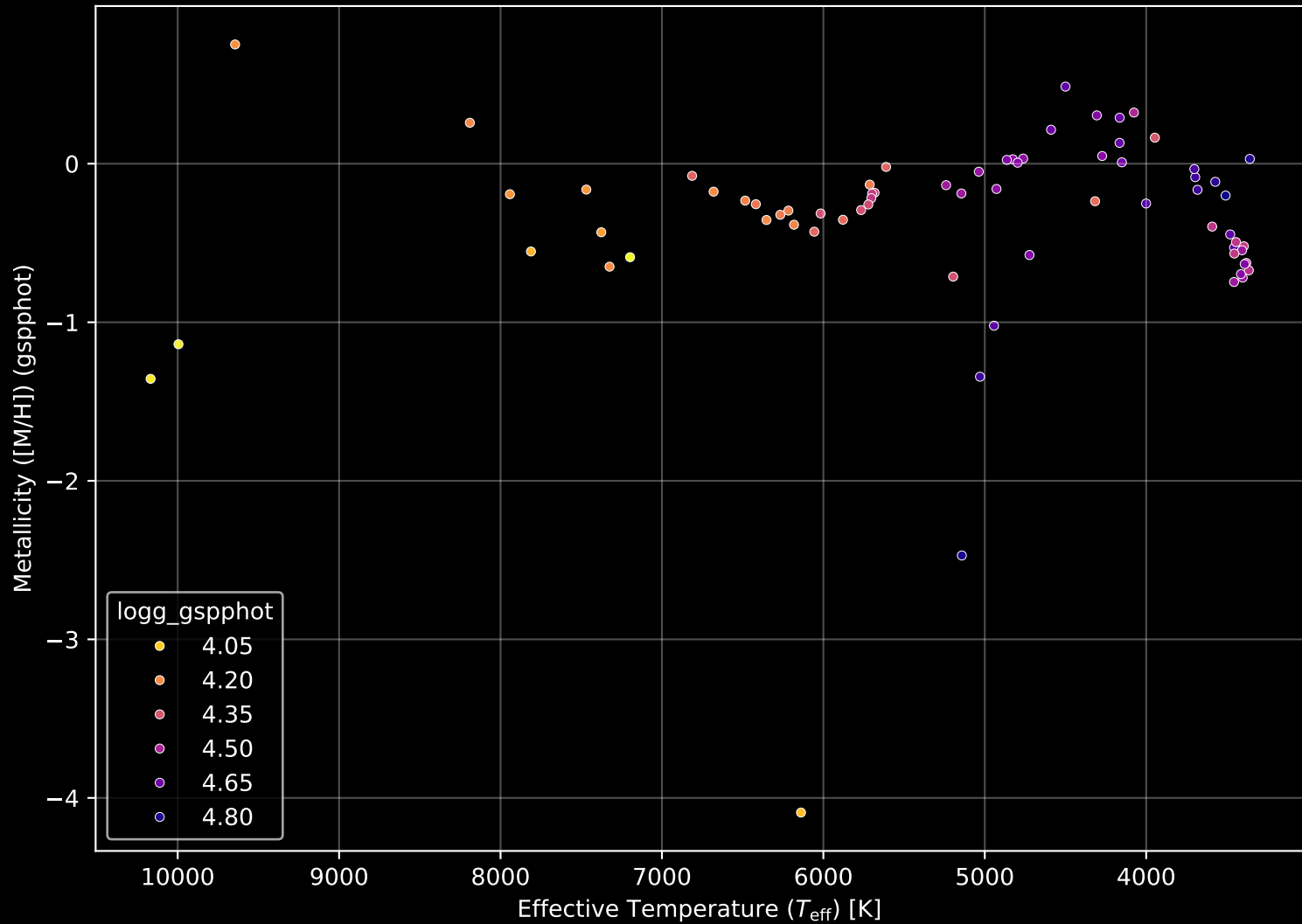
Gaia Cluster: [ASCC_101] Stellar Population Parameters (n= 72)
