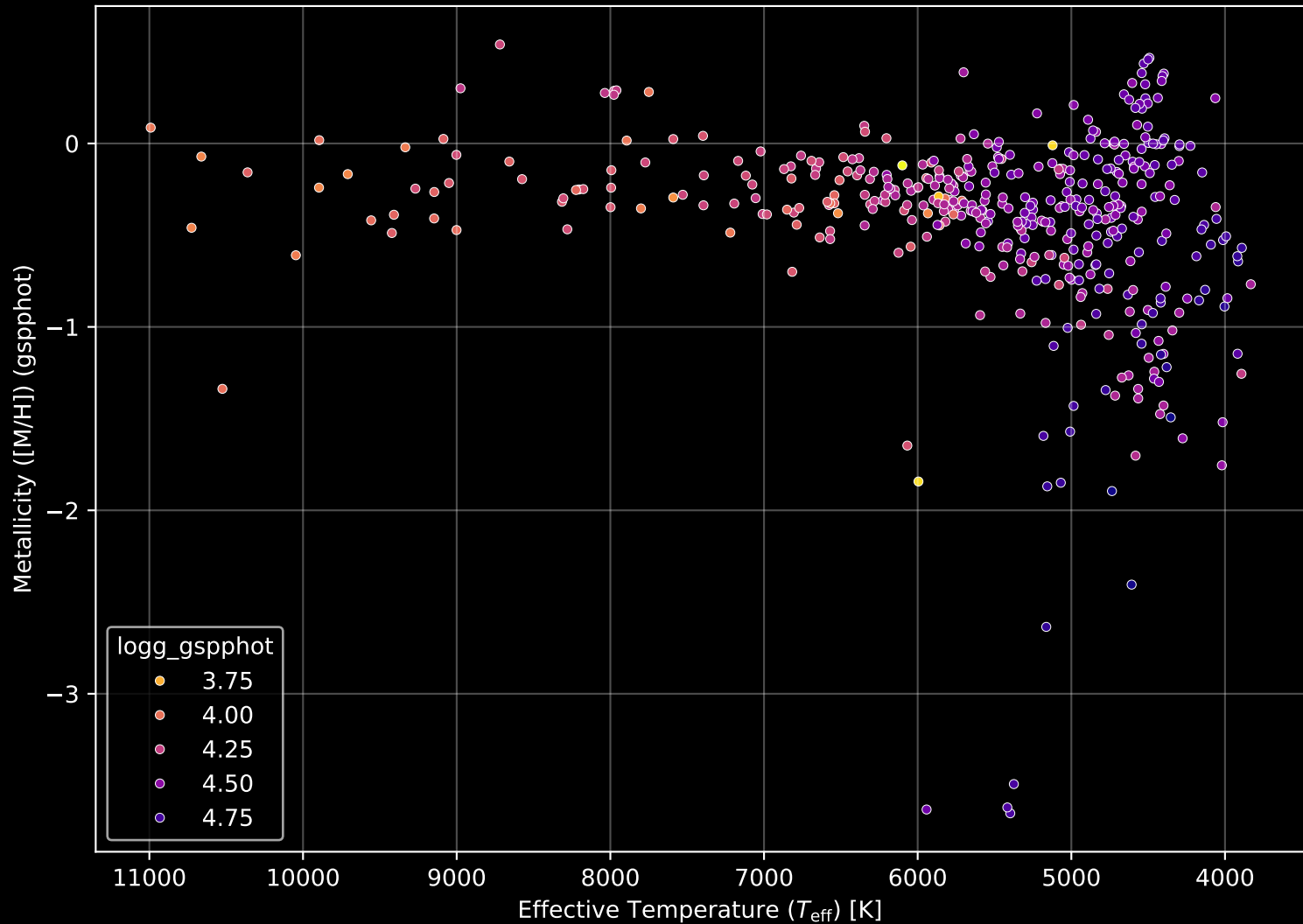
Gaia Cluster: [ASCC_108] Stellar Population Parameters (n= 439)
