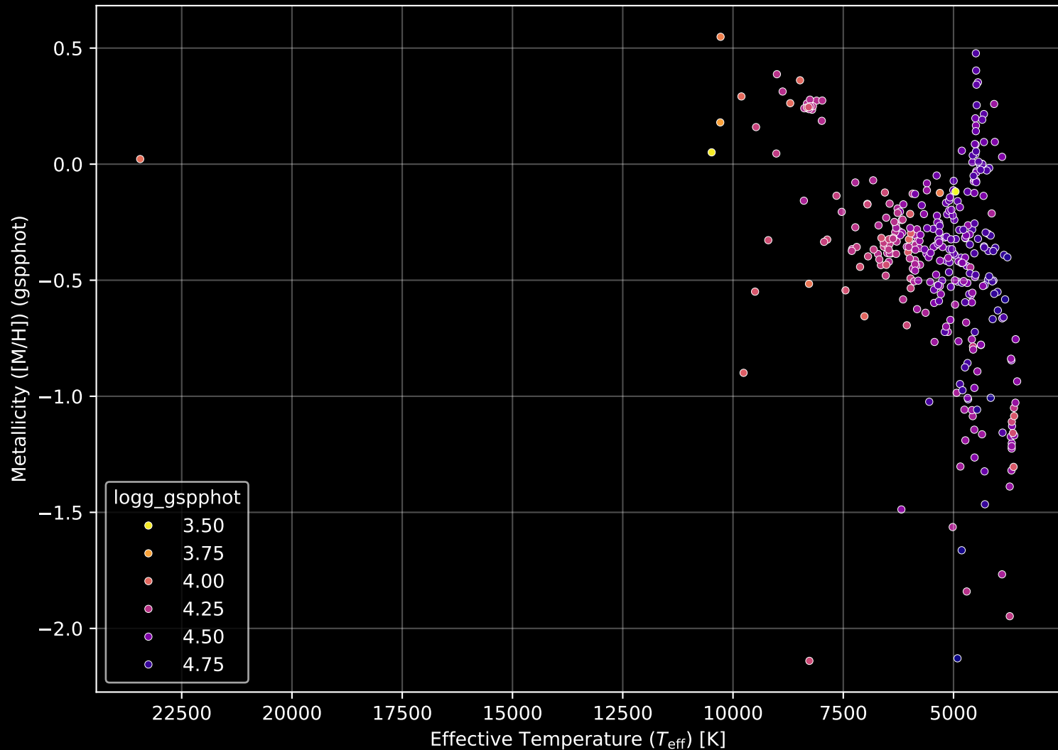
Gaia Cluster: [ASCC_11] Stellar Population Parameters (n= 339)
