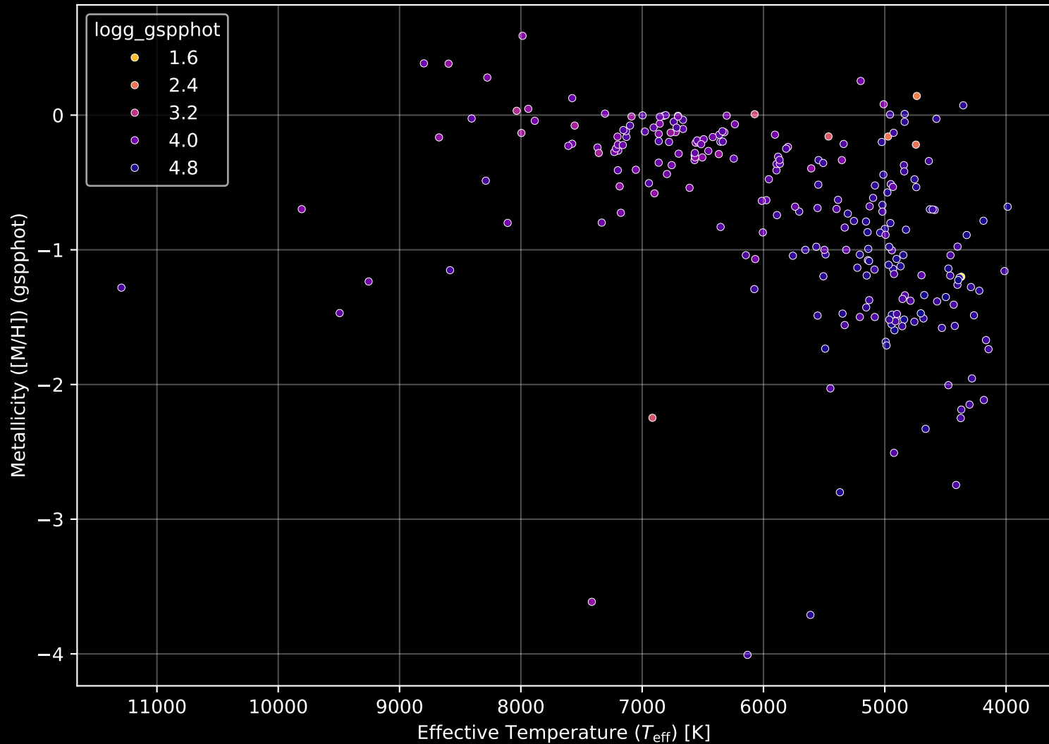
Gaia Cluster: [ASCC_110] Stellar Population Parameters (n= 241)
