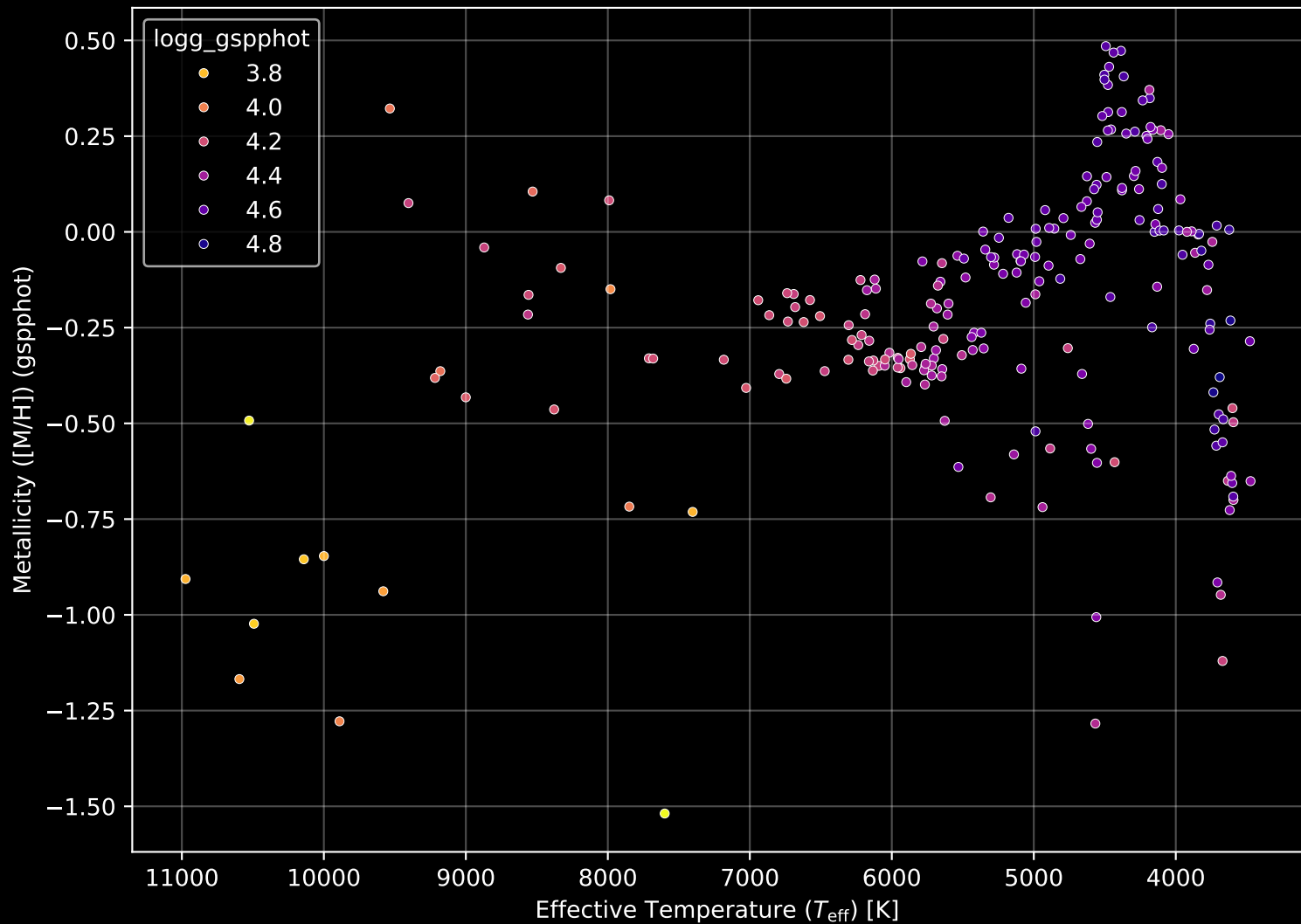
Gaia Cluster: [ASCC_113] Stellar Population Parameters (n= 229)
