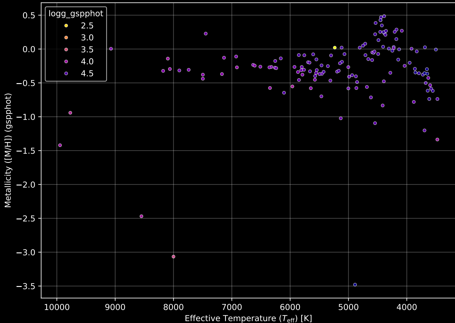
Gaia Cluster: [ASCC_23] Stellar Population Parameters (n= 136)
