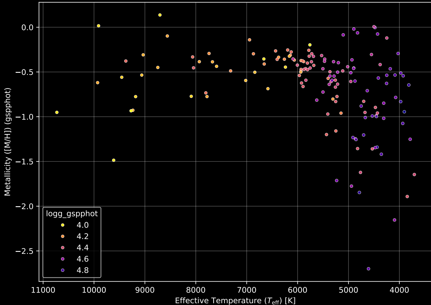
Gaia Cluster: [ASCC_30] Stellar Population Parameters (n= 151)
