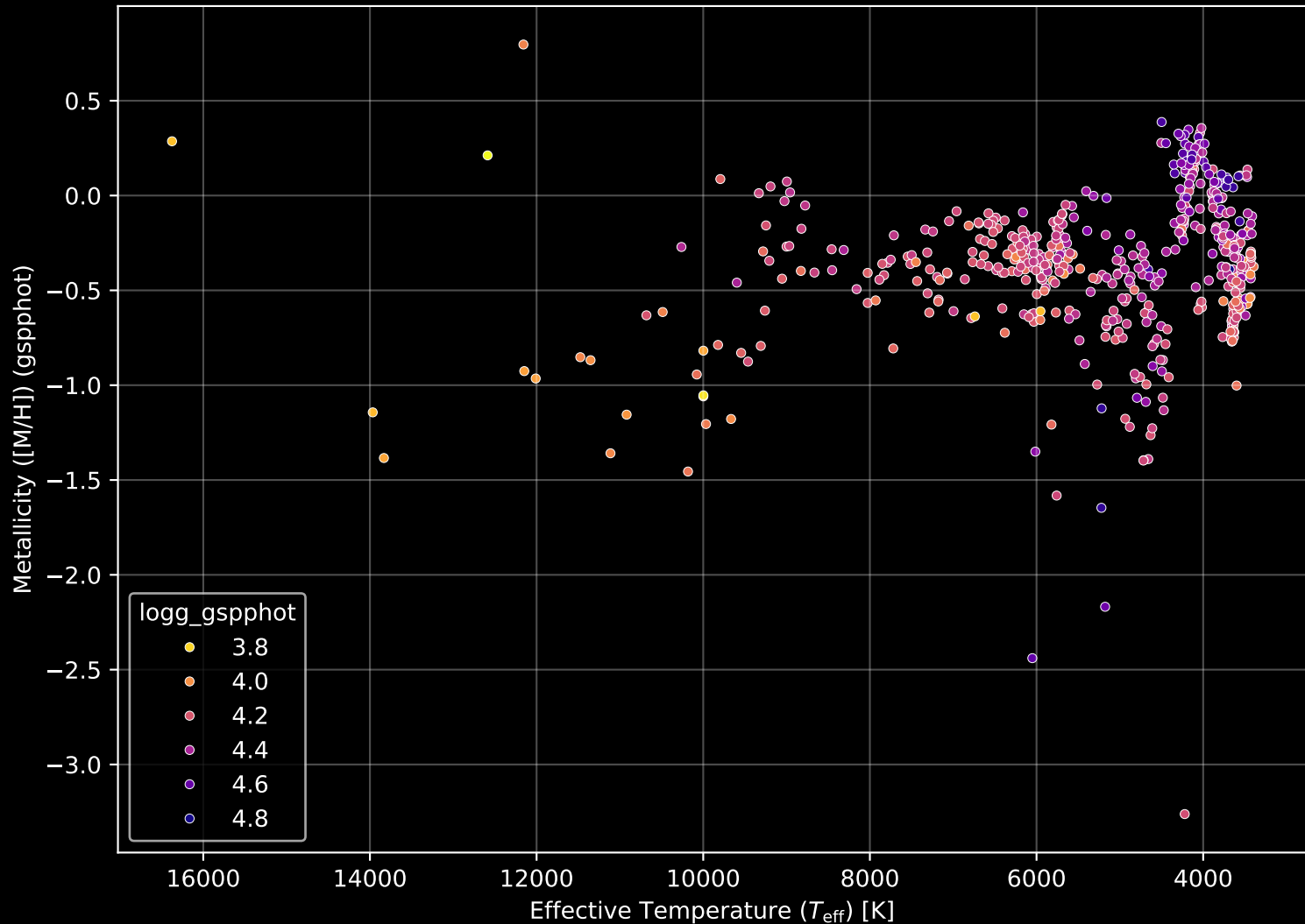
Gaia Cluster: [ASCC_32] Stellar Population Parameters (n= 553)
