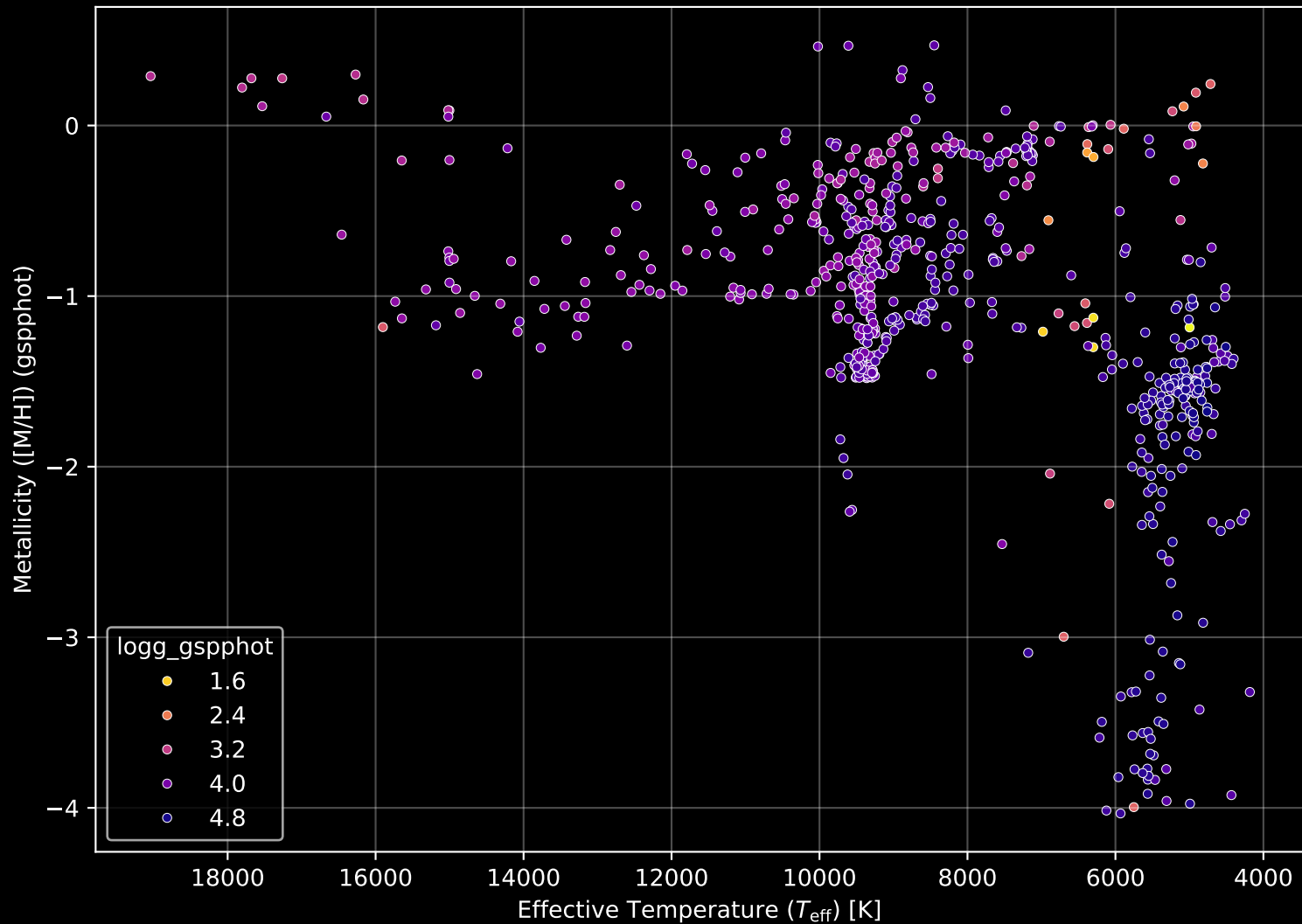
Gaia Cluster: [ASCC_9] Stellar Population Parameters (n= 711)
