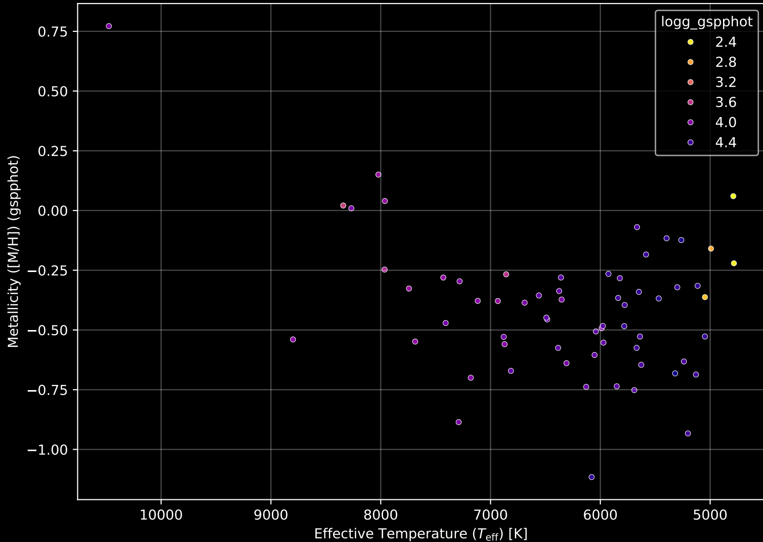
Gaia Cluster: [ASCC_90] Stellar Population Parameters (n= 63)
