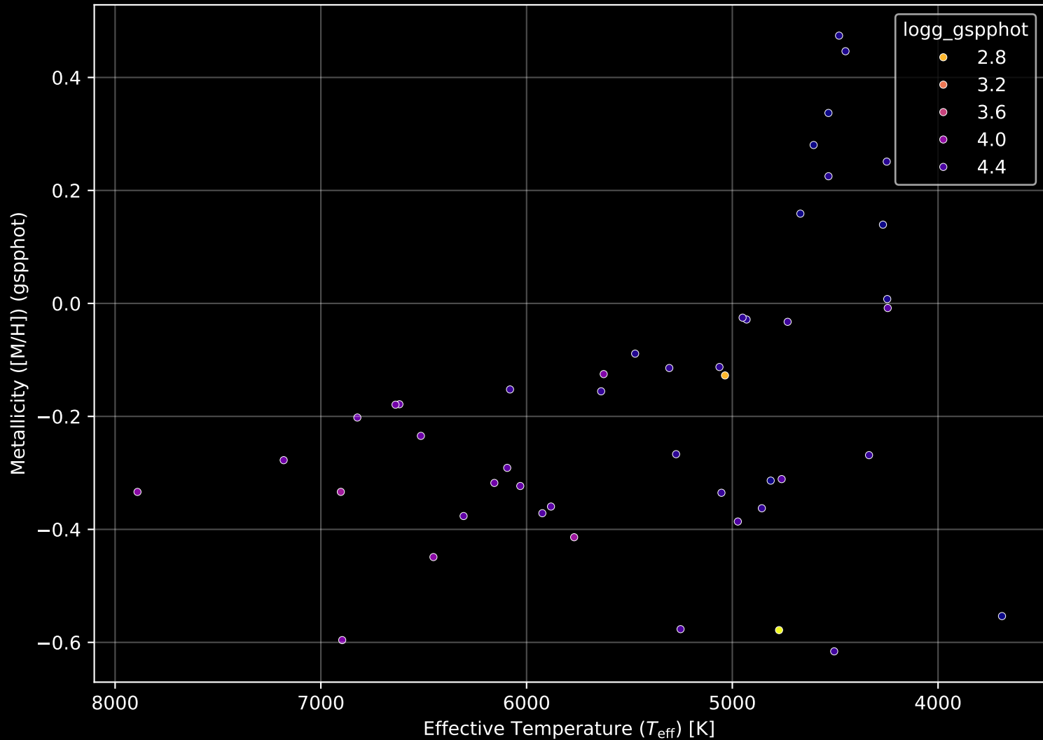
Gaia Cluster: [Alessi_1] Stellar Population Parameters (n= 47)
