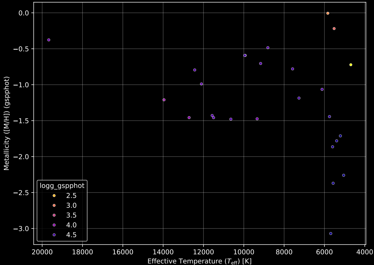
Gaia Cluster: [Alessi_18] Stellar Population Parameters (n= 26)
