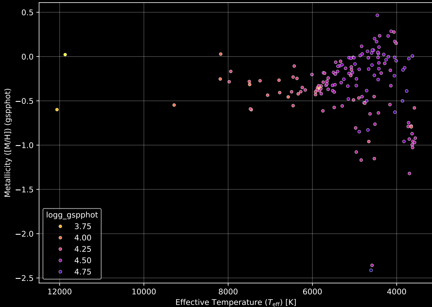
Gaia Cluster: [Alessi_37] Stellar Population Parameters (n= 158)
