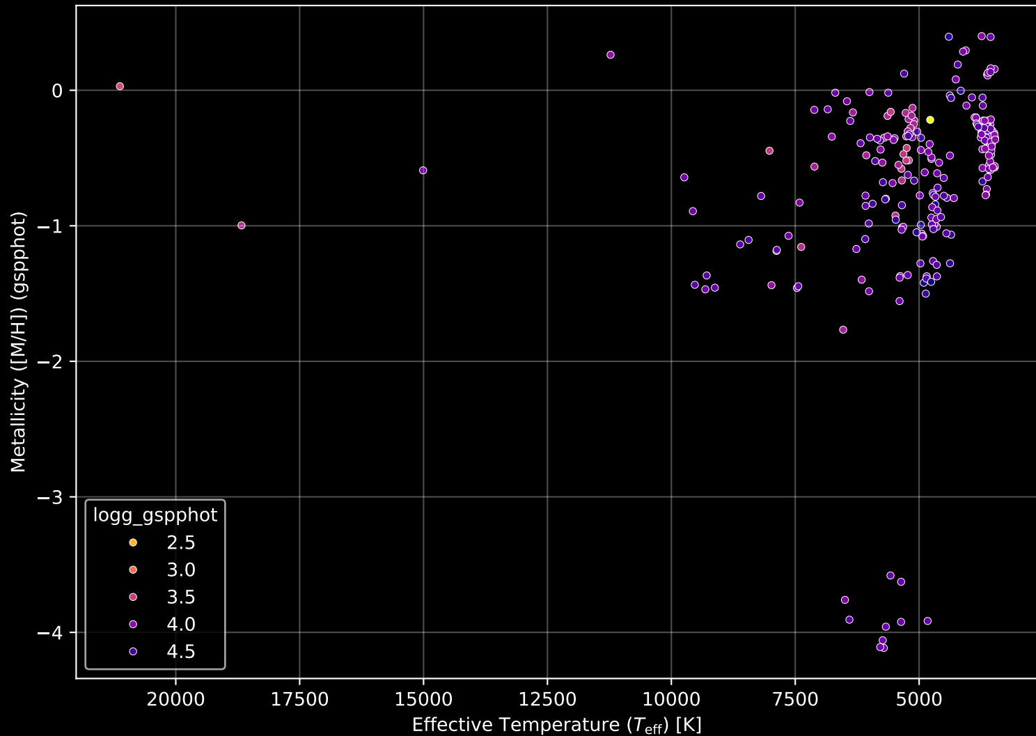
Gaia Cluster: [Alessi_43] Stellar Population Parameters (n= 258)
