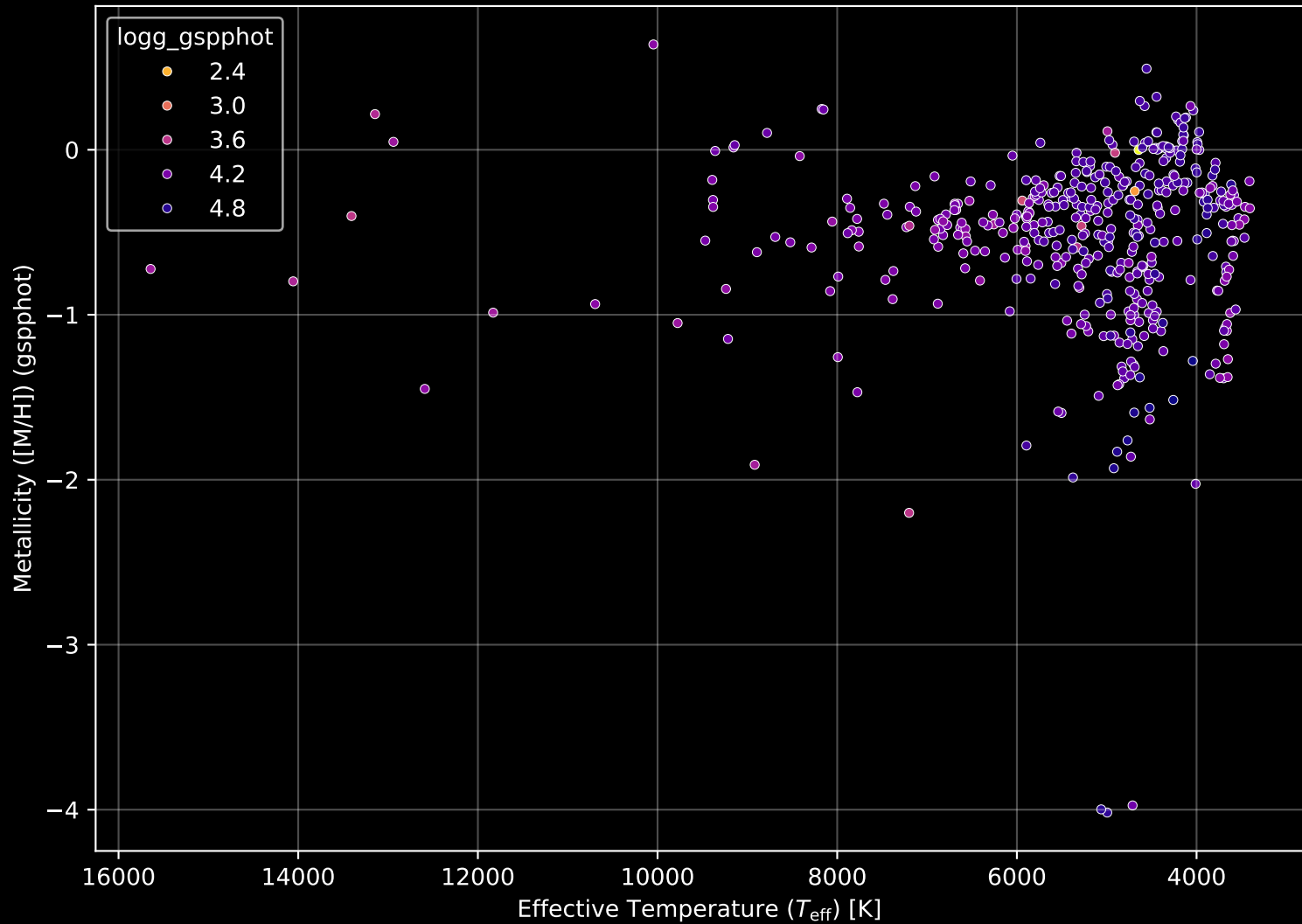
Gaia Cluster: [Alessi_44] Stellar Population Parameters (n= 454)
