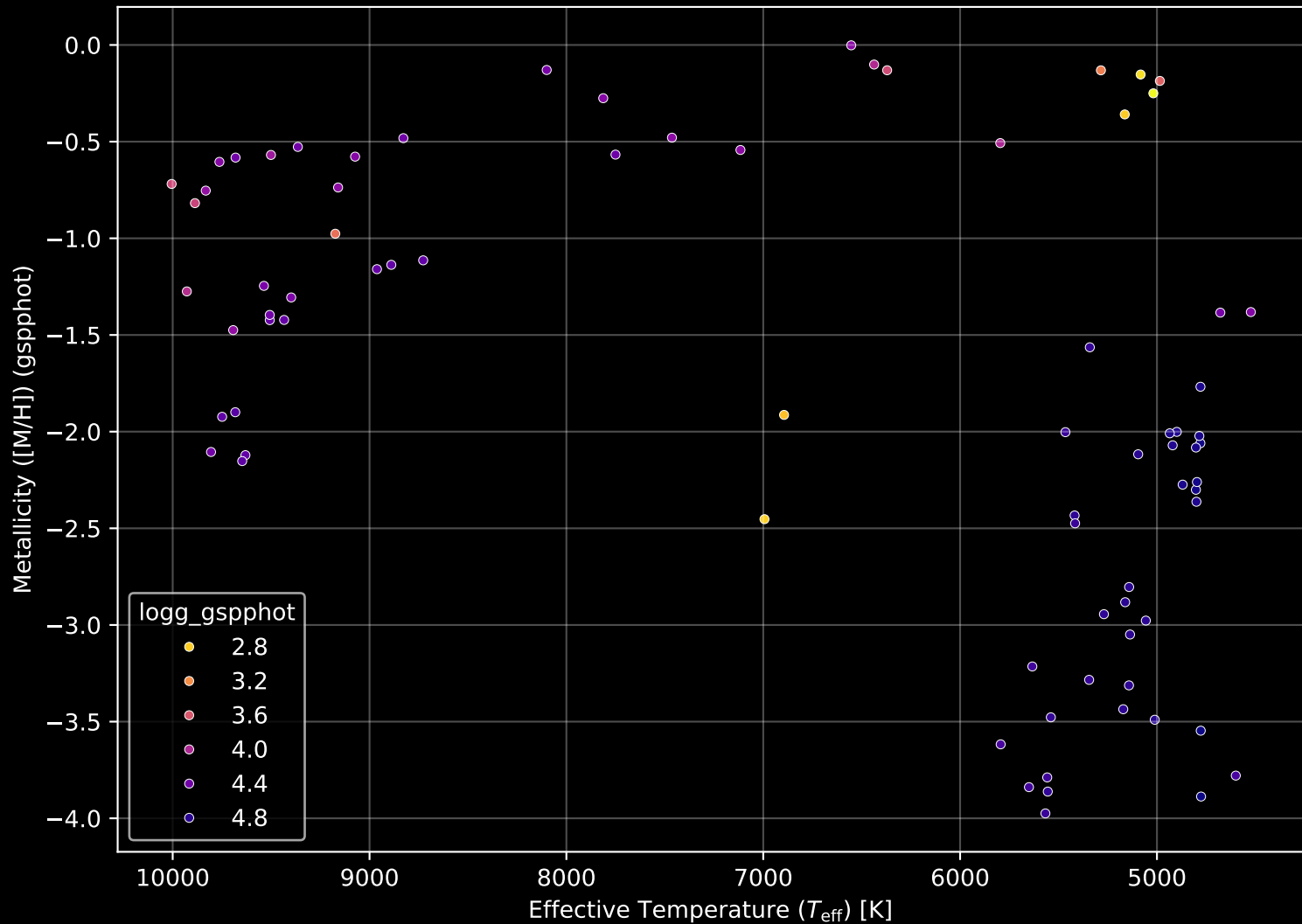
Gaia Cluster: [Alessi_53] Stellar Population Parameters (n= 79)
