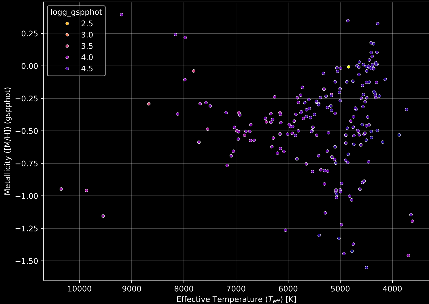
Gaia Cluster: [Alessi_6] Stellar Population Parameters (n= 207)
