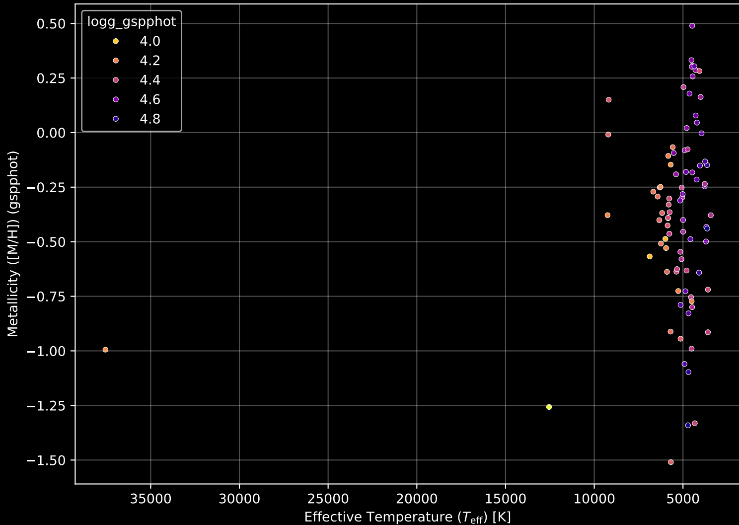
Gaia Cluster: [Alessi_Teutsch_12] Stellar Population Parameters (n= 87)
