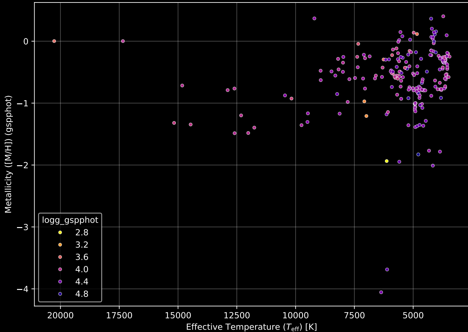
Gaia Cluster: [Alessi_Teutsch_5] Stellar Population Parameters (n= 228)
