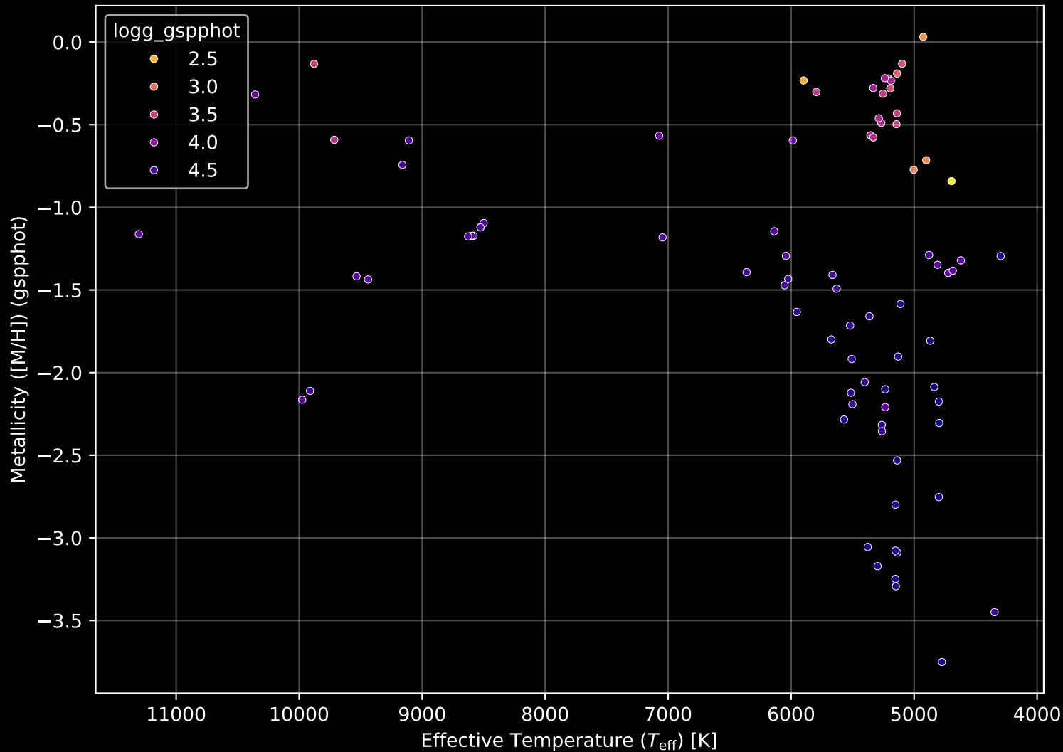
Gaia Cluster: [Auner_1] Stellar Population Parameters (n= 82)
