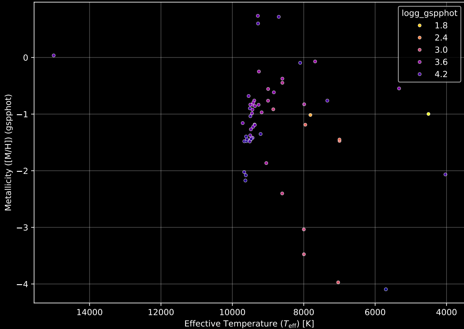
Gaia Cluster: [BH_37] Stellar Population Parameters (n= 59)
