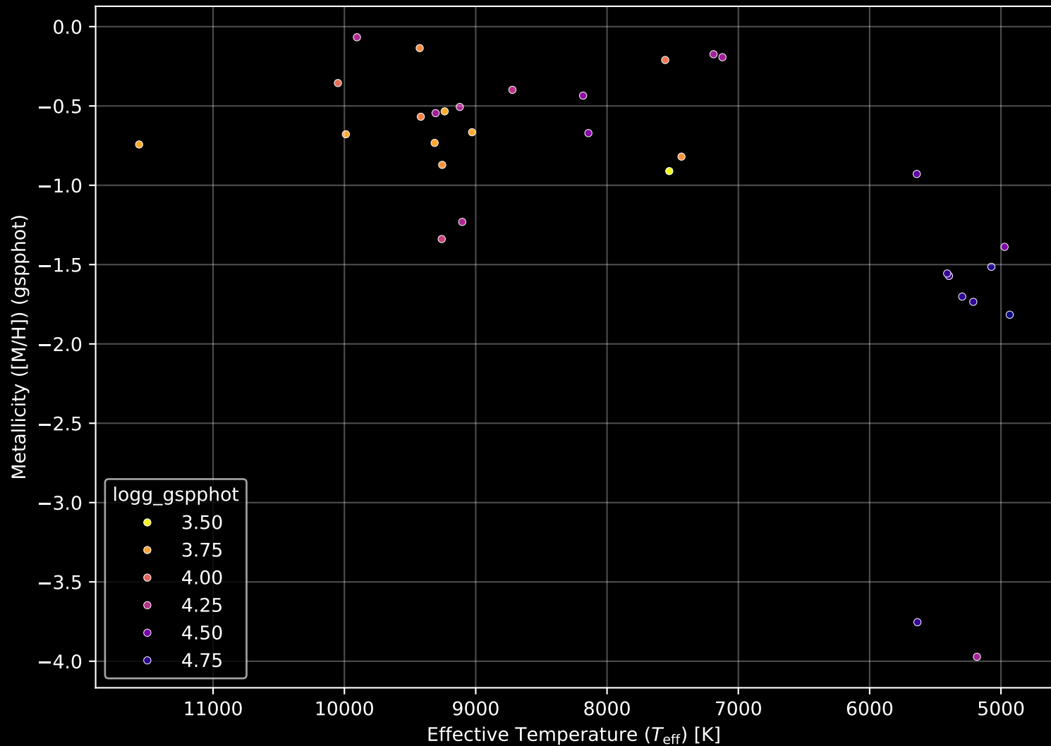
Gaia Cluster: [Basel_10] Stellar Population Parameters (n= 32)
