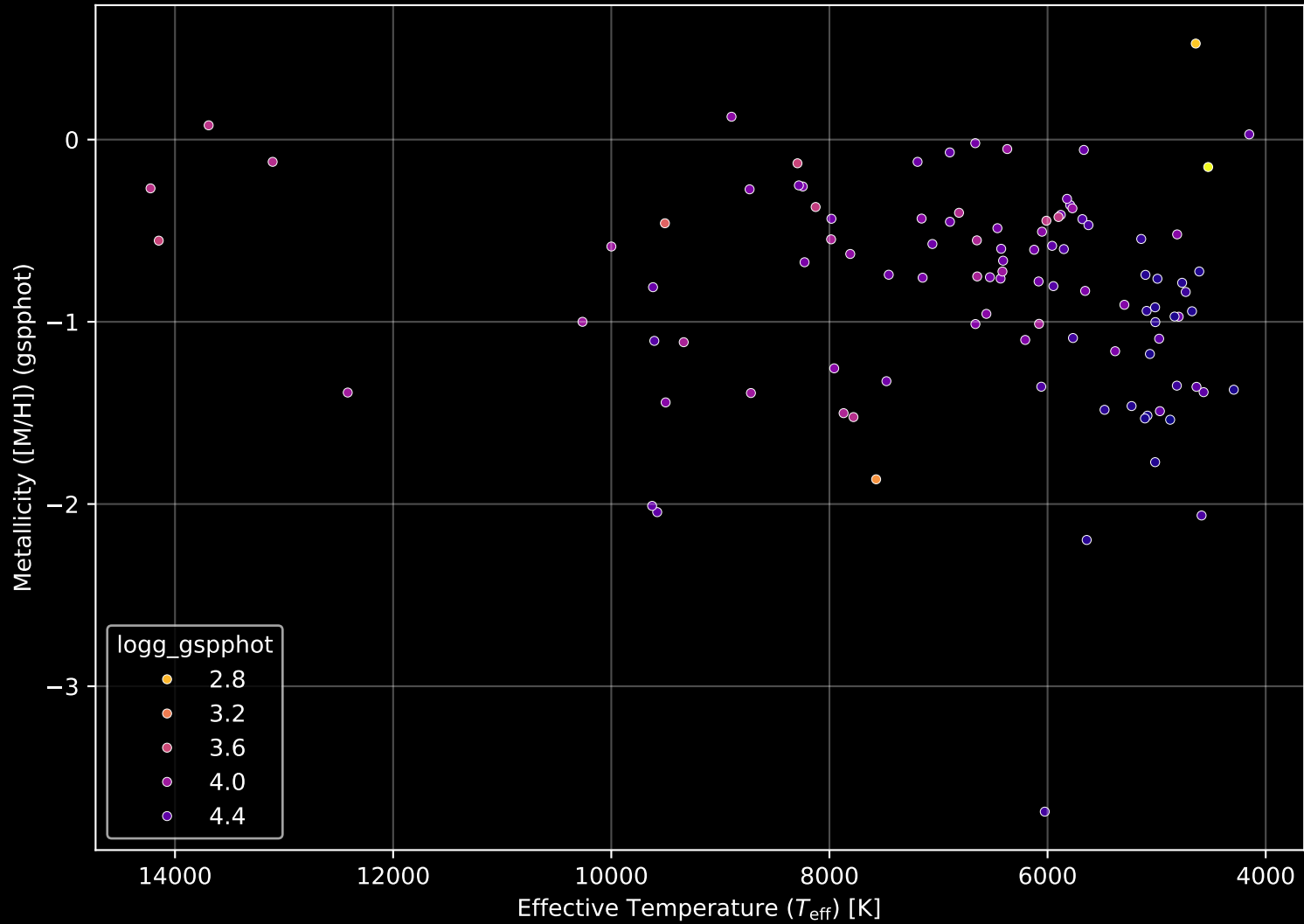
Gaia Cluster: [Basel_18] Stellar Population Parameters (n= 104)
