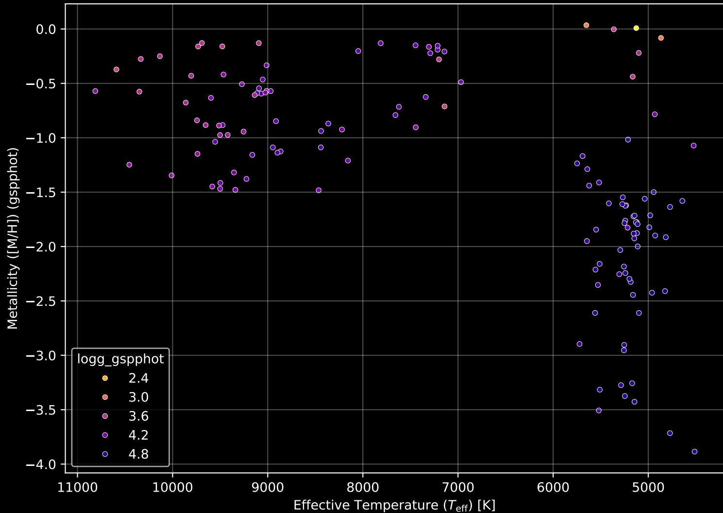
Gaia Cluster: [Basel_4] Stellar Population Parameters (n= 132)
