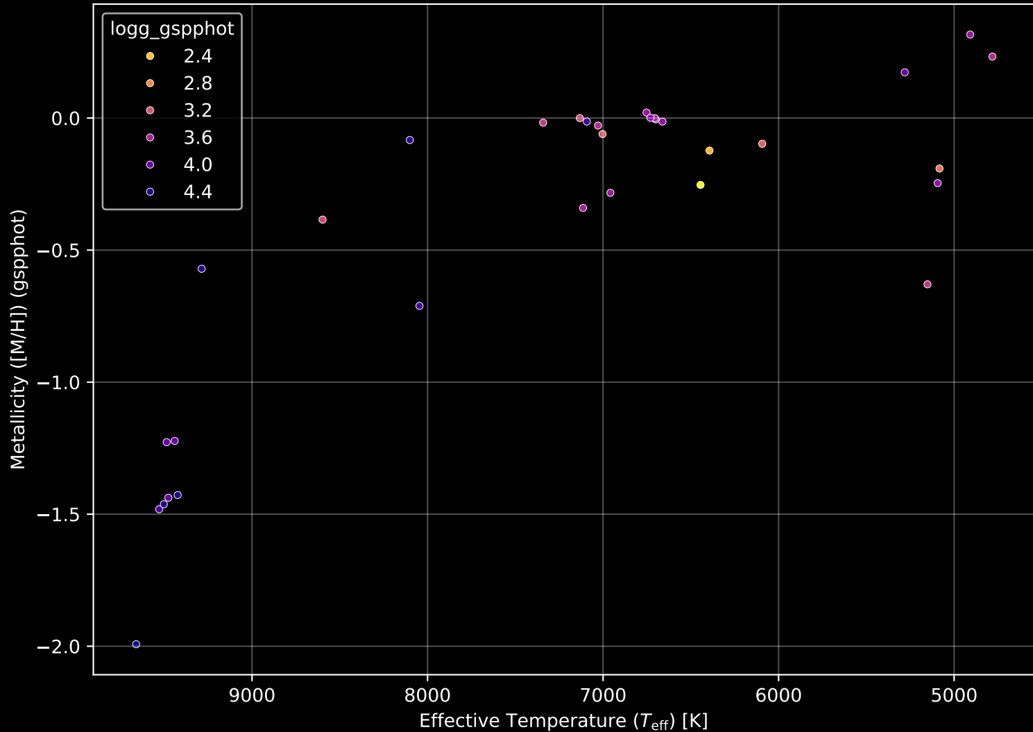
Gaia Cluster: [Berkeley_103] Stellar Population Parameters (n= 32)
