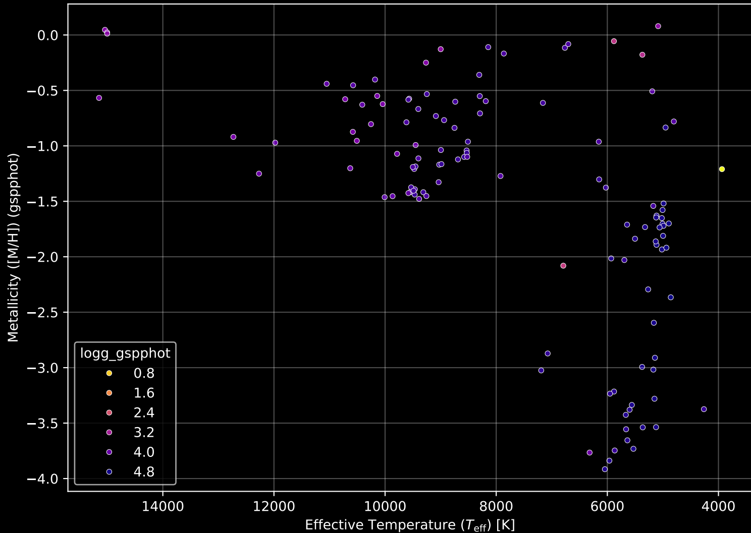
Gaia Cluster: [Berkeley_11] Stellar Population Parameters (n= 121)
