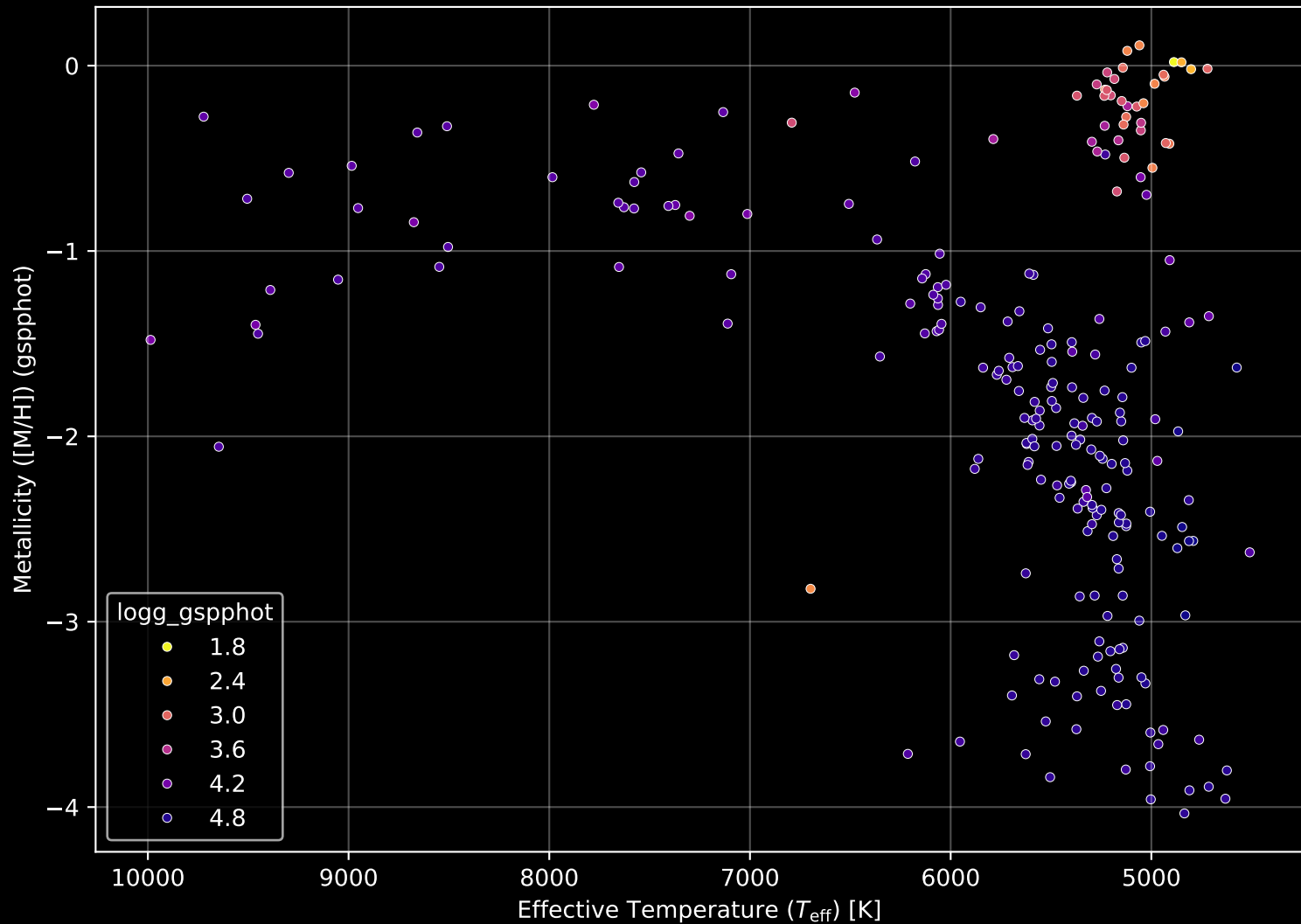
Gaia Cluster: [Berkeley_14] Stellar Population Parameters (n= 239)
