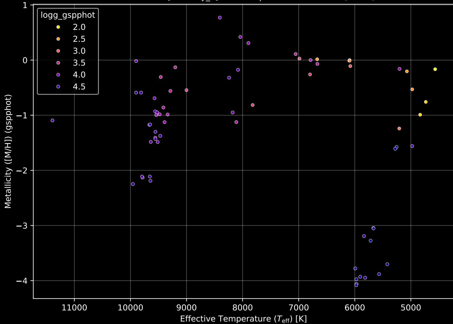
Gaia Cluster: [Berkeley_2] Stellar Population Parameters (n= 69)
