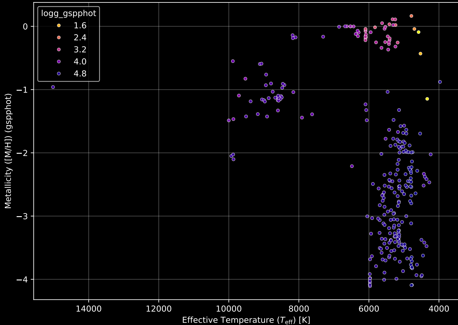
Gaia Cluster: [Berkeley_24] Stellar Population Parameters (n= 285)
