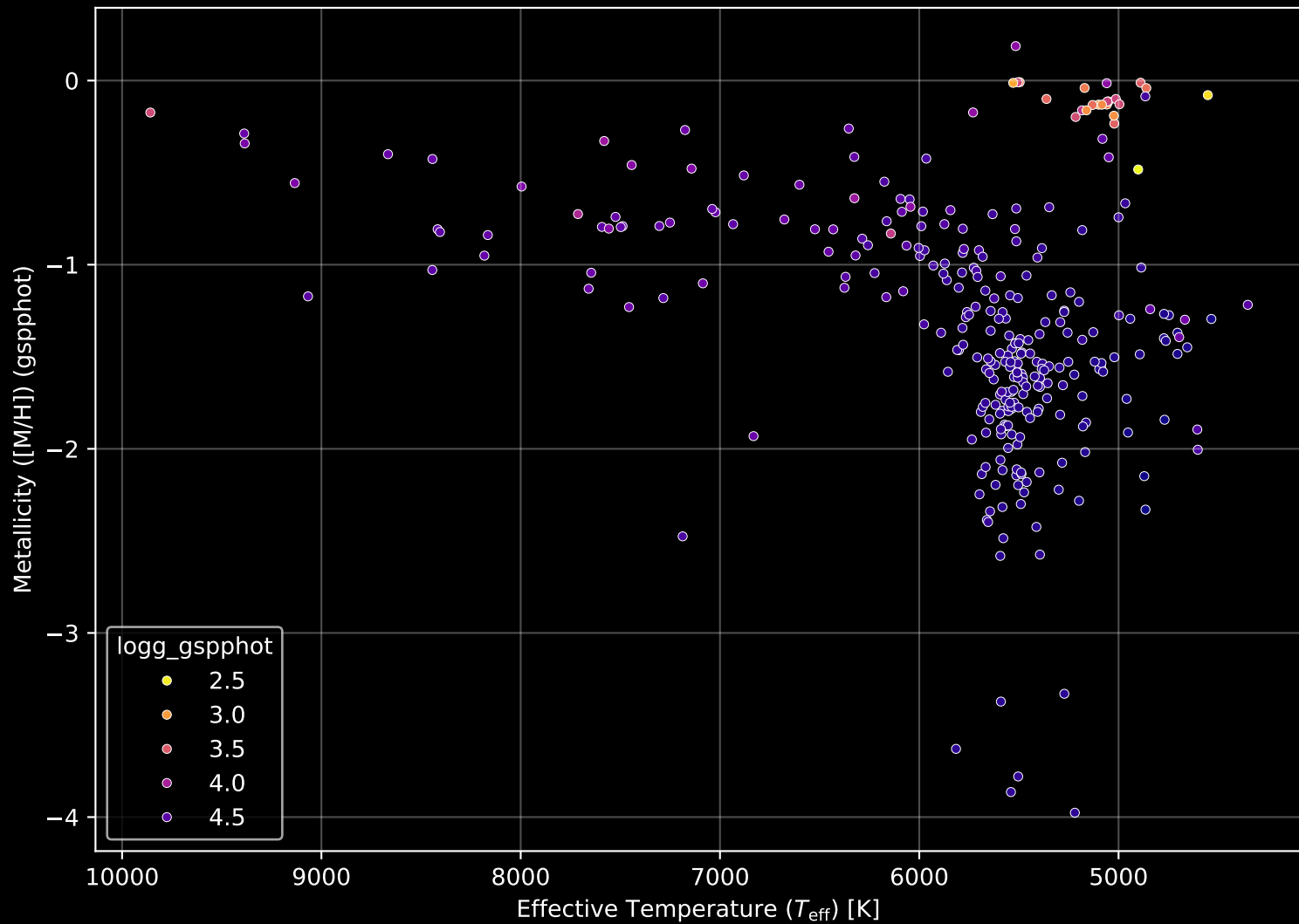
Gaia Cluster: [Berkeley_31] Stellar Population Parameters (n= 303)
