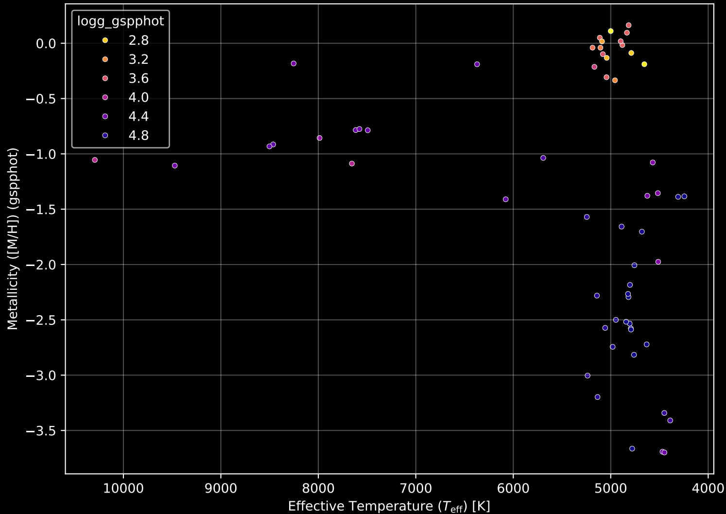
Gaia Cluster: [Berkeley_34] Stellar Population Parameters (n= 59)
