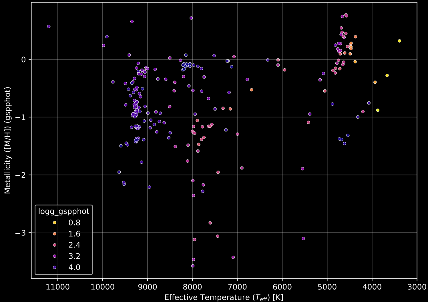
Gaia Cluster: [Berkeley_43] Stellar Population Parameters (n= 226)
