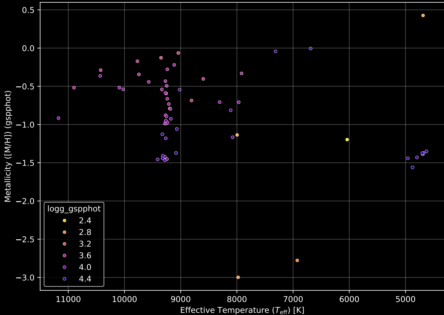
Gaia Cluster: [Berkeley_47] Stellar Population Parameters (n= 64)
