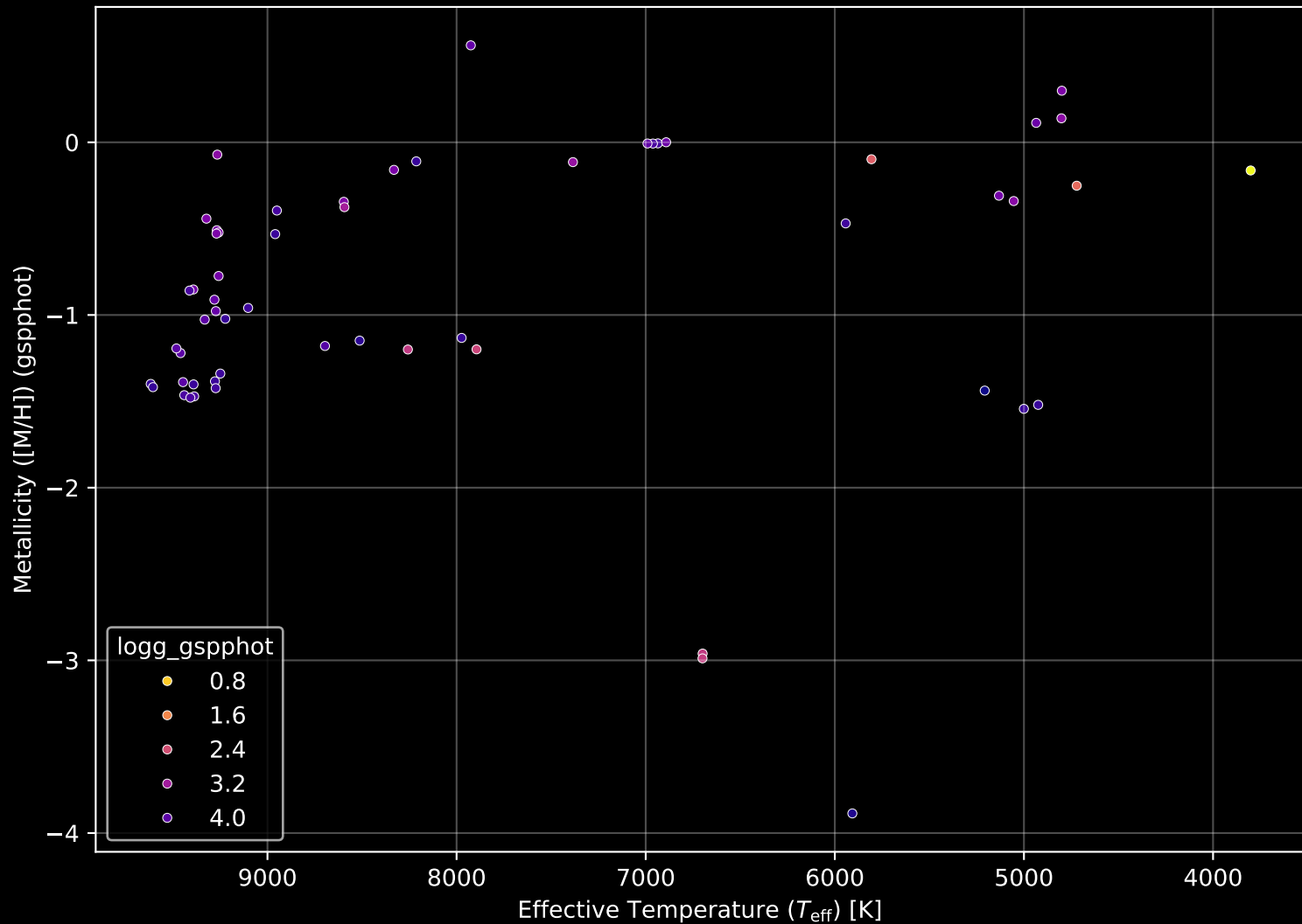
Gaia Cluster: [Berkeley_49] Stellar Population Parameters (n= 57)
