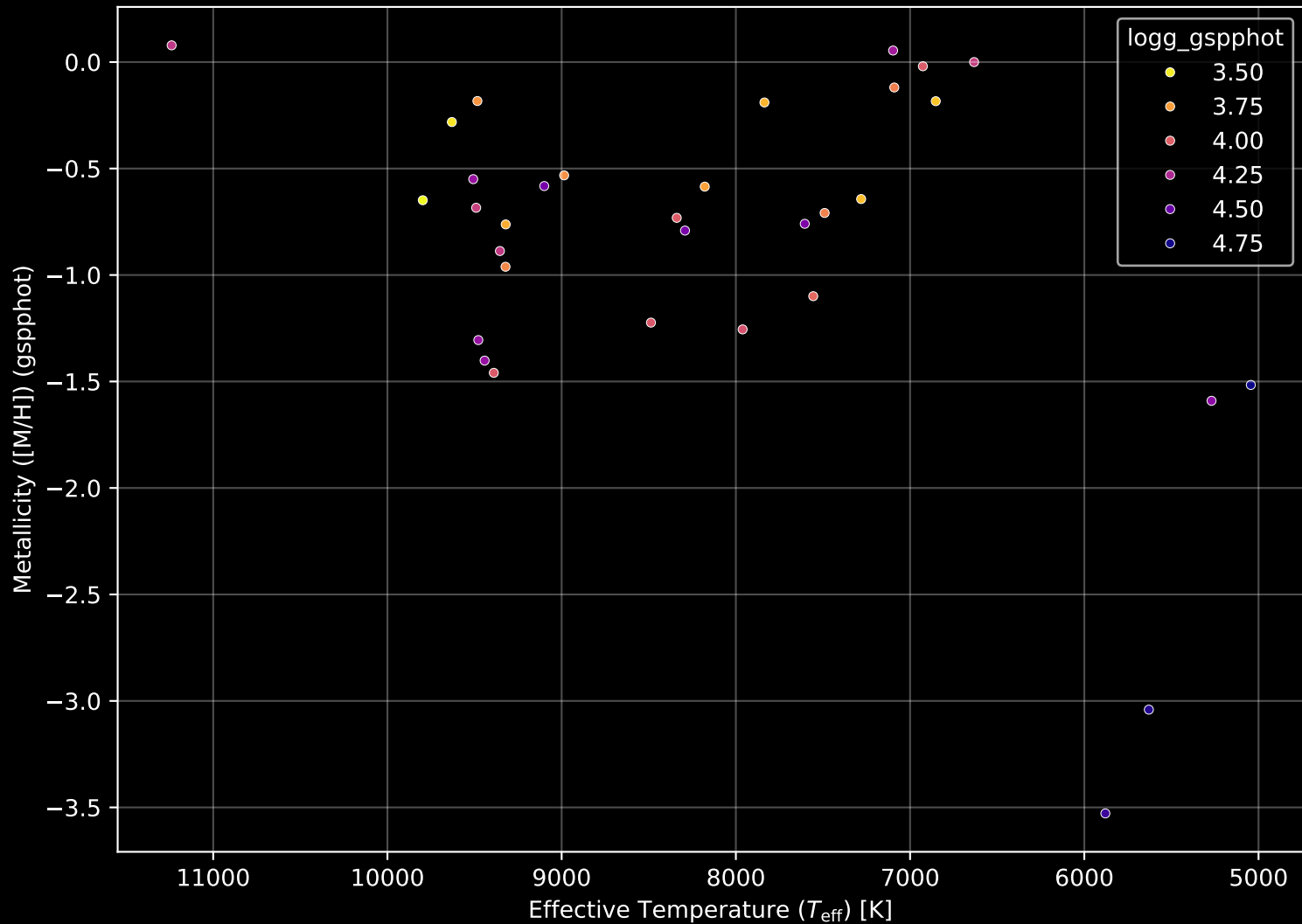
Gaia Cluster: [Berkeley_5] Stellar Population Parameters (n= 33)
