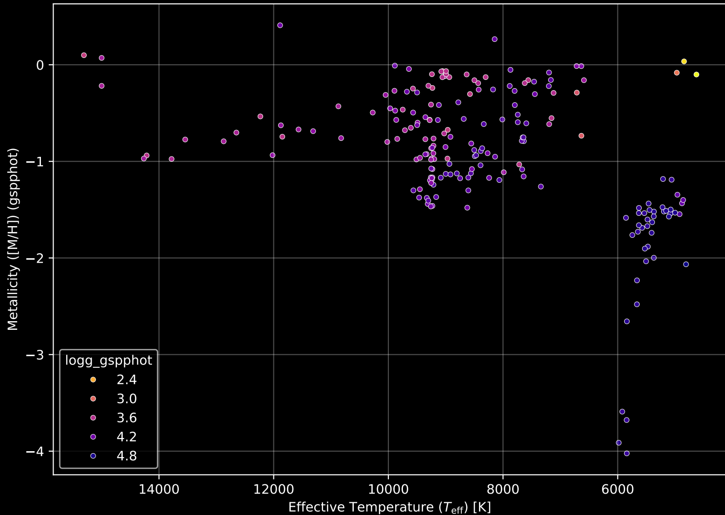
Gaia Cluster: [Berkeley_6] Stellar Population Parameters (n= 198)
