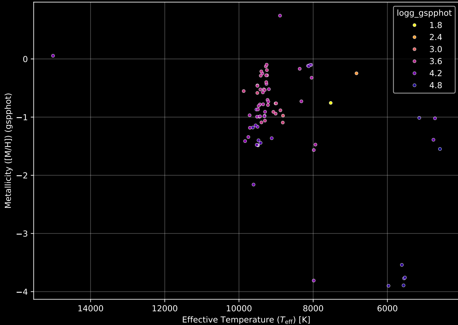
Gaia Cluster: [Berkeley_60] Stellar Population Parameters (n= 80)
