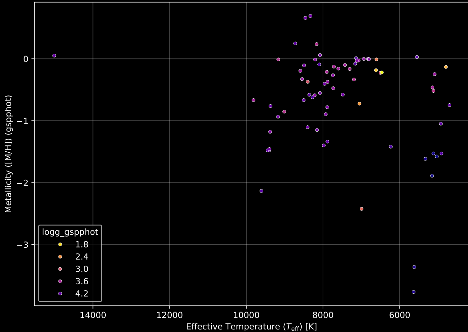
Gaia Cluster: [Berkeley_66] Stellar Population Parameters (n= 72)
