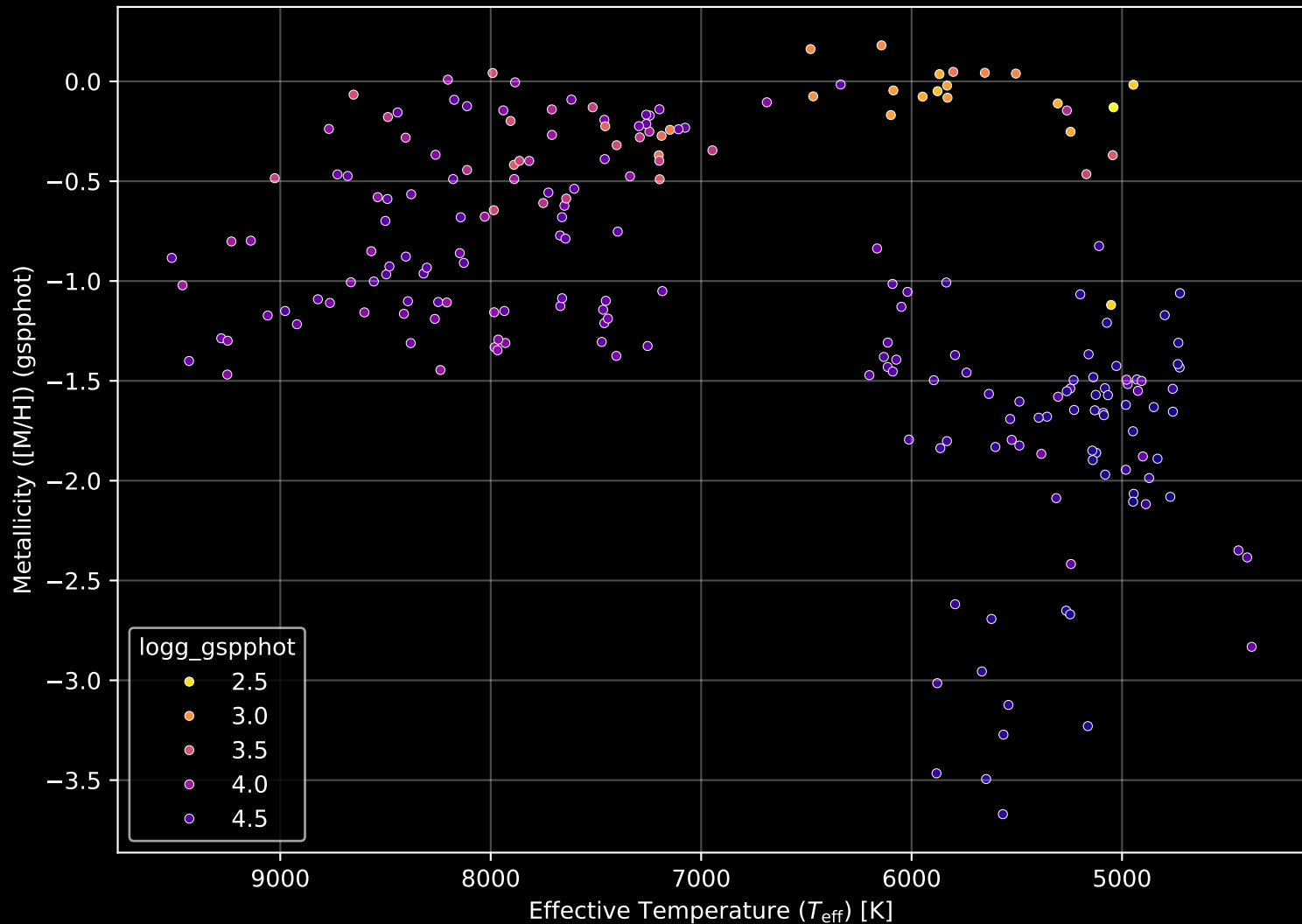
Gaia Cluster: [Berkeley_67] Stellar Population Parameters (n= 219)
