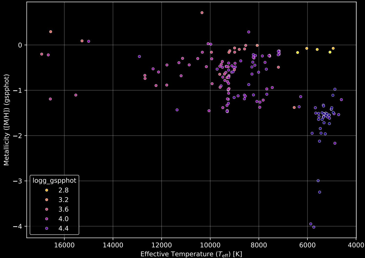
Gaia Cluster: [Berkeley_7] Stellar Population Parameters (n= 170)
