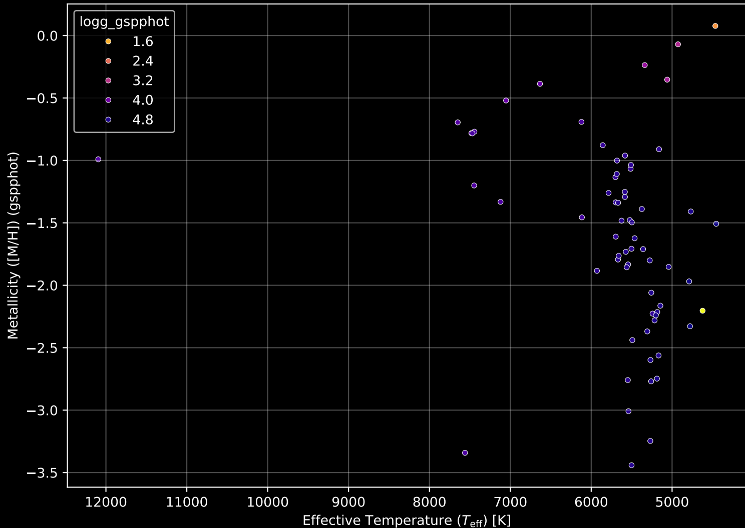
Gaia Cluster: [Berkeley_73] Stellar Population Parameters (n= 66)
